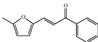
3-(5-Methylfuran-2-yl)-1-phenylprop-2-en-1-one
