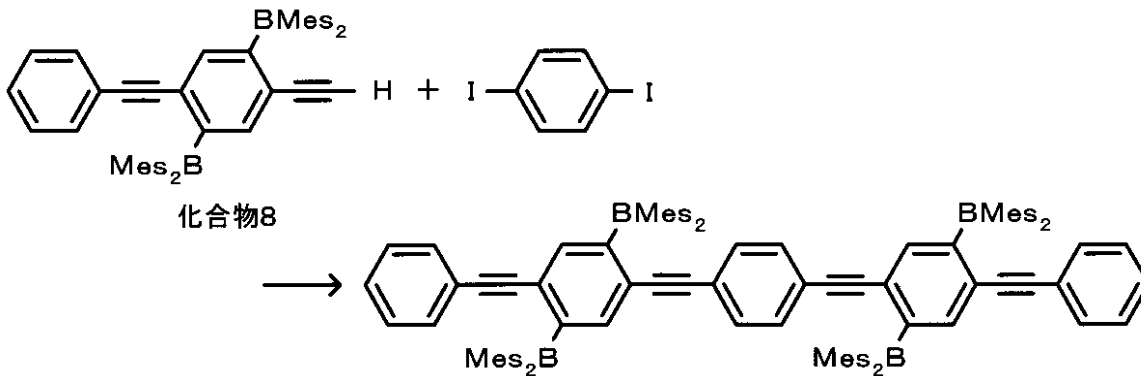
化合物9
