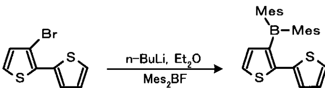
化合物21
