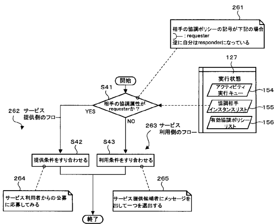
S14の協議候補から協議する相手を決定する処理を示すフローチャート
