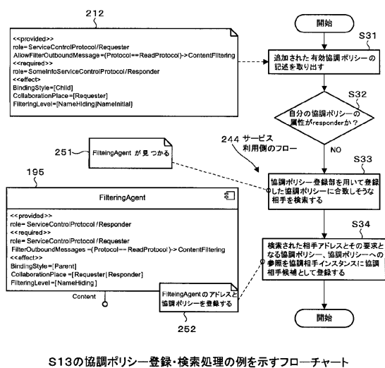
S13の協議ポリシー登録・検索処理の例を示すフローチャート
