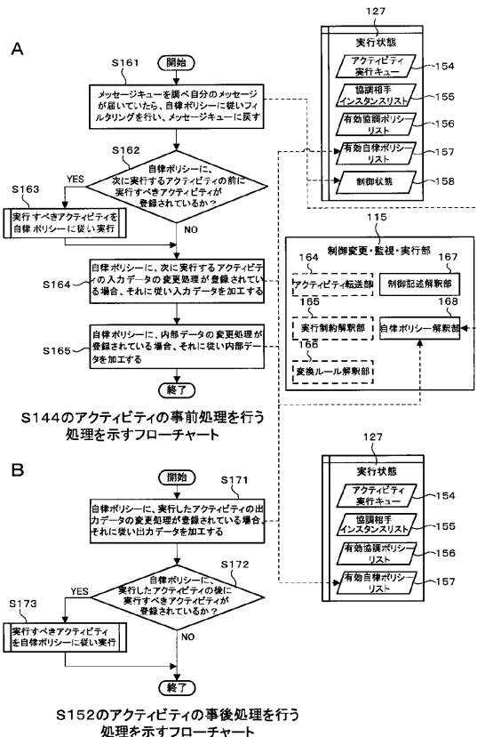
S152のアクティビティの事後処理を行う処理を示すフローチャート
