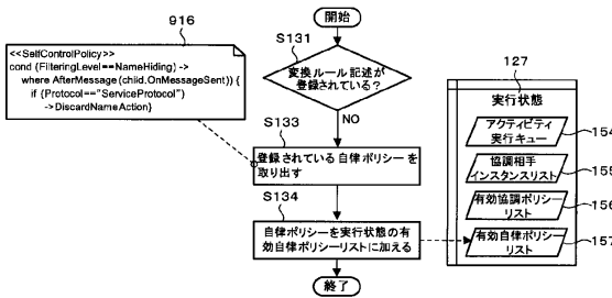
S18の自律ポリシー選択・生成・登録処理の例(FilteringAgent)を示すフローチャート
