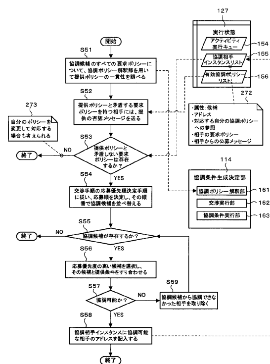
S42の提供条件のすり合わせで協議候補サービスを提供する相手を決定する処理を示すフローチャート
