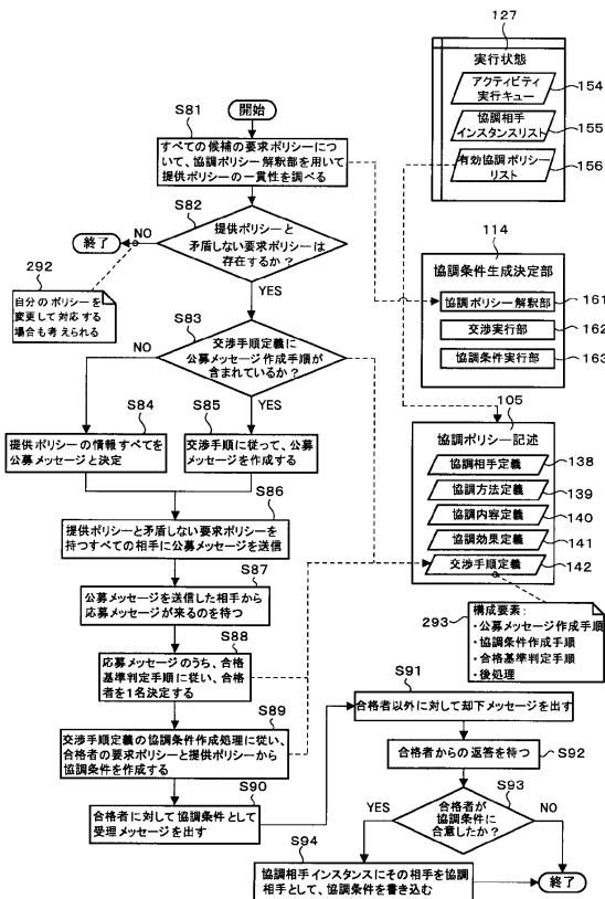
S43の利用条件のすり合わせで協調候補からサービスを利用する相手を決する処理を示すフローチャート
