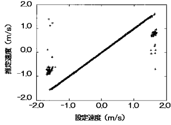
(c) 本発明に係る広帯域ドプラ法
