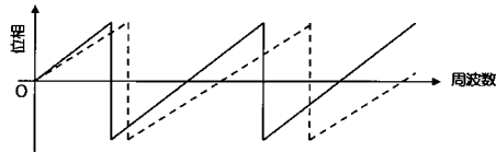
(d) 受波スペクトルの位相差
