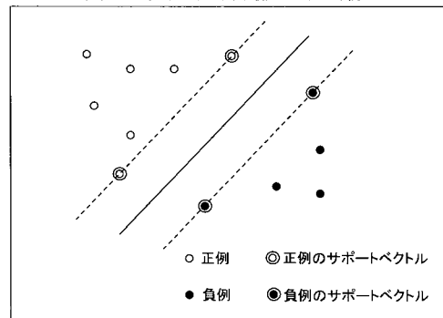
サポートベクトルマシンの最大マージンの例
