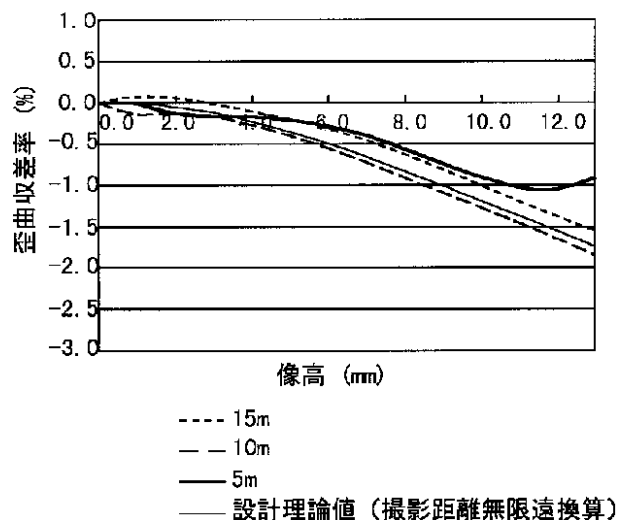
各撮影距離ごとの歪曲収差率の分布 (%)
