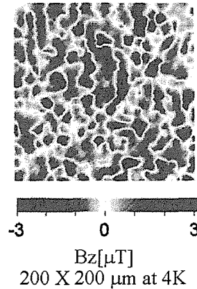
[図] Co(5.8%)ドーブしたTiO 2 の磁区構造
