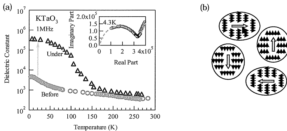
第2図 (a) \text{KTaO}_3 における光誘起巨大分極形成。光を当てると赤から青に誘電率が2桁増大する。挿入図はその分散をCole-Coleプロットしたもの。 (b) 光誘起強誘電マイクロドメインモデル。光励起キャリアを中心に強誘電ドメインが形成される。
