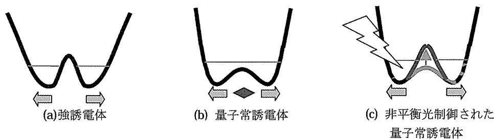
第1図 強誘電体(a)、量子常誘電体(b)の局所ポテンシャル。量子常誘電体においては、零点振動のため秩序(図の右向きまたは左向き矢印)が形成されない。非平衡光制御により量子常誘電体の局所ポテンシャルを(a)に変形すれば強誘電体が形成されると期待される(c)。
