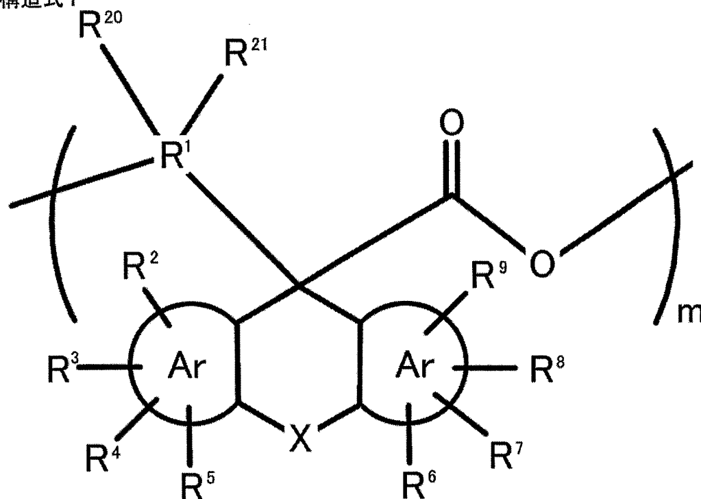
構造式1
