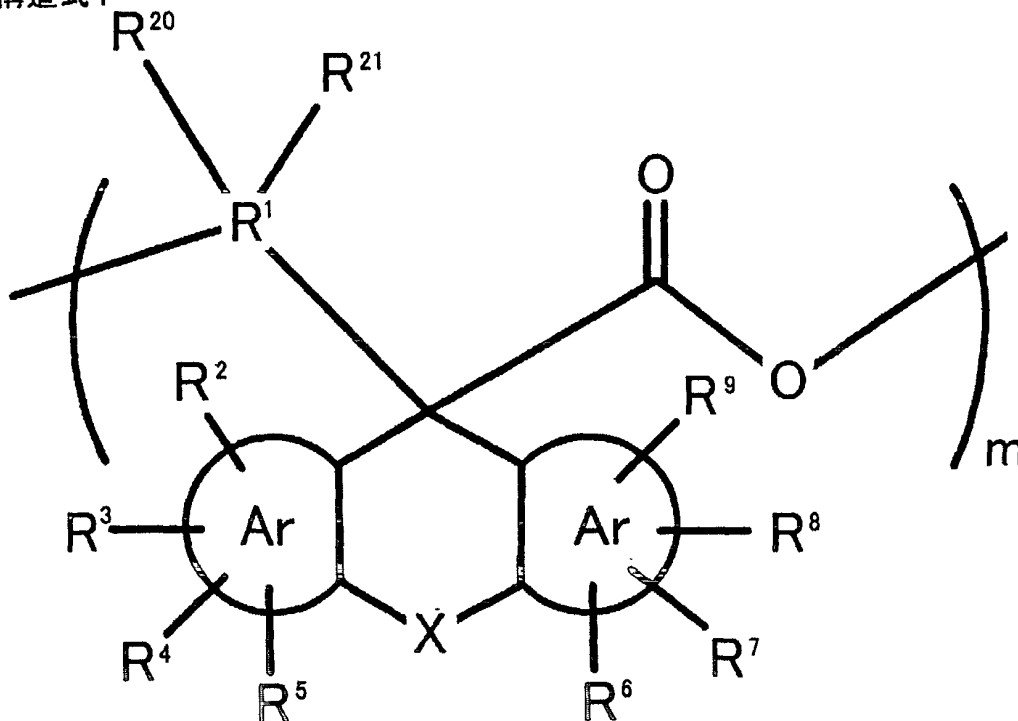
構造式1
