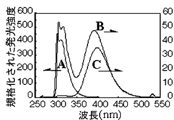
フルオレン(A), ジベンジフルベンオリゴマー(二量体(B), 三量体～17量体混合物(C))のTHF中室温(約23度)での蛍光スペクトル。吸収強度は濃度 1.0 \times 10^{-5} Mに規格化した。[励起波長265 nm(A), 267 nm(B,C)]
