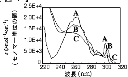
フルオレン(A), ジベンジフルベンオリゴマー(二量体(B), 三量体～17量体混合物(C))のTHF中室温(約23度)での吸収スペクトル
