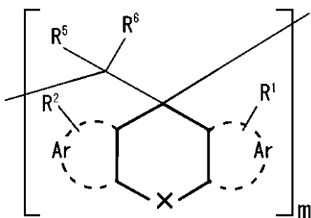
構造式 1
