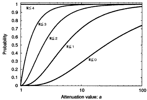
減衰値の補正値 a に対する周辺の無線通信局数の確率分布
