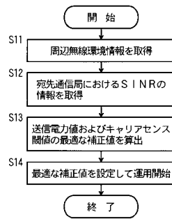
無線通信局の処理手順例
