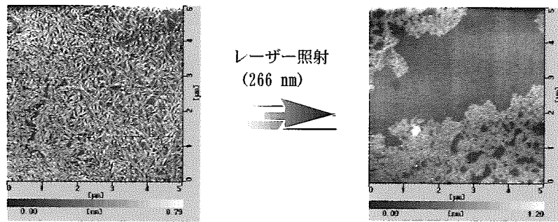
図1 マイカ基板上に形成したフィブロインの2次元超薄膜（左）。ランダムコイル型のペプチド鎖が基板上に2次元ネットワークを形成している。これに266 nm レーザー光を照射すると、 \beta シート型アイランド状に転移する（右）。
