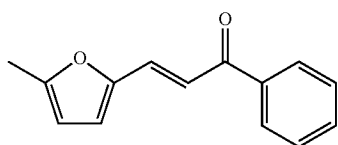
3-(5-Methylfuran-2-yl)-1-phenylprop-2-en-1-one
