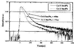
図2 GSOの発光減衰曲線 (蛍光減衰時間：Ce濃度0.5mol%、1.5mol%それぞれ60ns、35ns)
