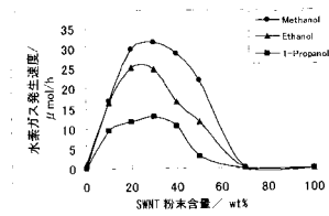
SWNT含量を変化させたときの水素ガス発生速度のアルコールの種類への依存性 (T1 O 2 粉末とSWNT粉末の合計全量: 30mg, アルコール濃度: 50vol%, にそれぞれ固定した)
