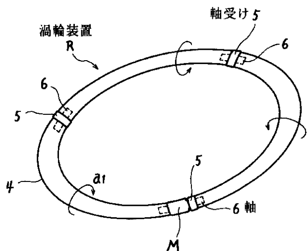
渦輪の軸受け構造
