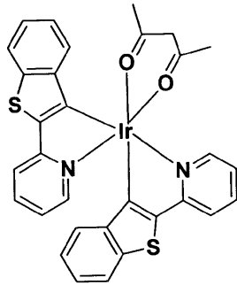
BTP 2 Ir(acac)
