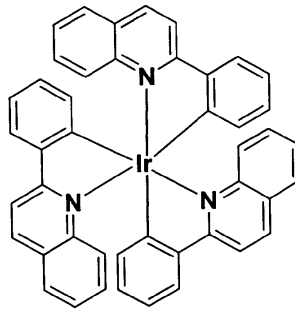
PQ 3 Ir
