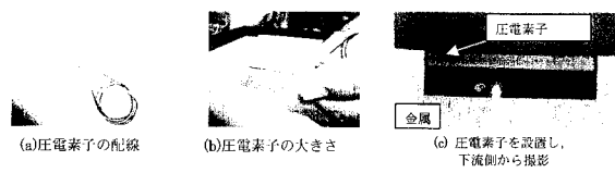
図3 圧電素子の写真
