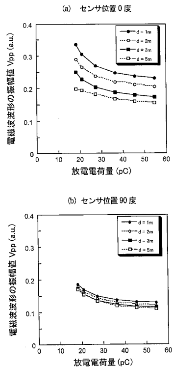
電磁波振幅値 V_{pp} と放電電荷量の関係
