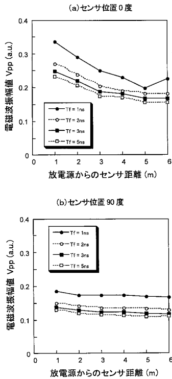
電磁波振幅値 V_{pp} のセンサ距離およびセンサ位置依存性
