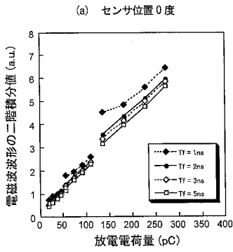
電磁波波形の二階積分値と放電電荷量の関係
