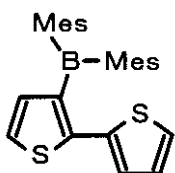
化合物22
