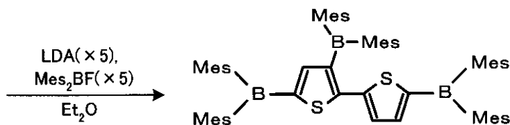
化合物24
