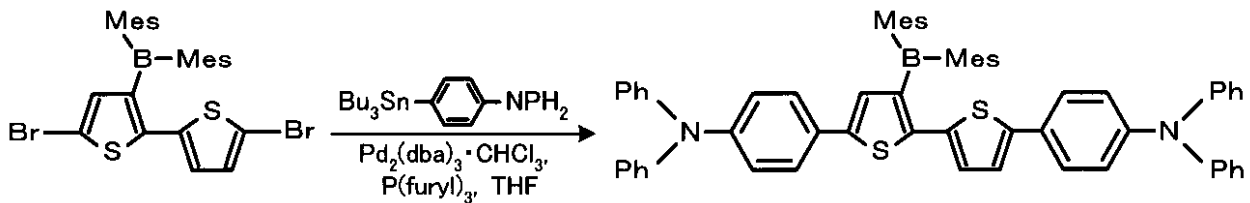
化合物25
