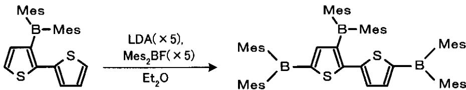
化合物22
