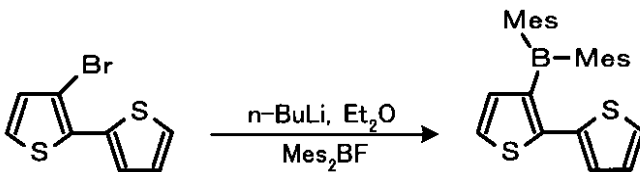
化合物21
