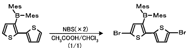
化合物22
