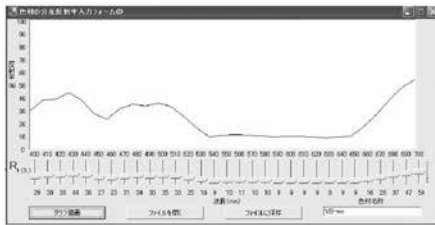
バジターブルーとNanoTek Powderの1対1混合の分光反射率
