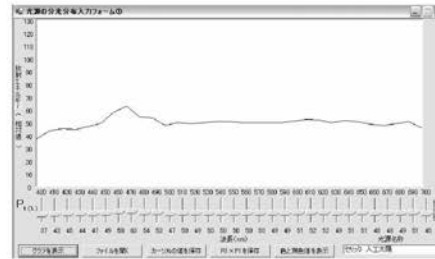
シリック人工太陽の分光分布
