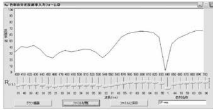
シェルビングとNanoTek Powderの1対1混合の分光反射率
