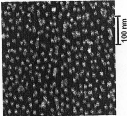
(b) 成長途中の金ナノ薄膜(150秒成長)
