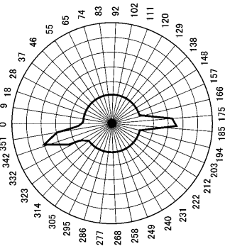
(b) ハンガ一角度360° の際の頭部圧力分布
