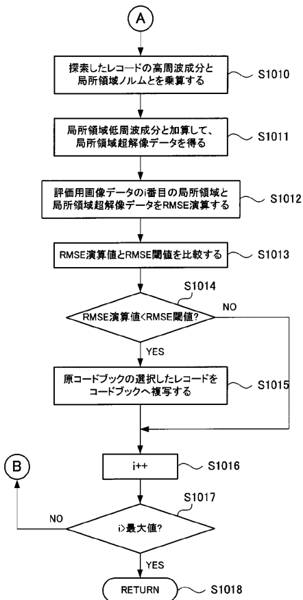
レコード選定処理(後半)
