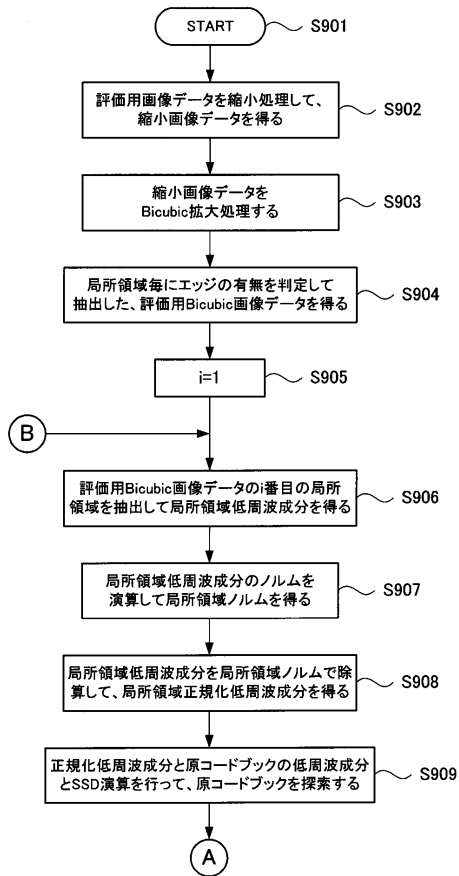
レコード選定処理(前半)
