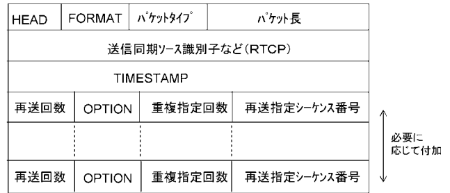
NACK-RTCPパケットの構成
