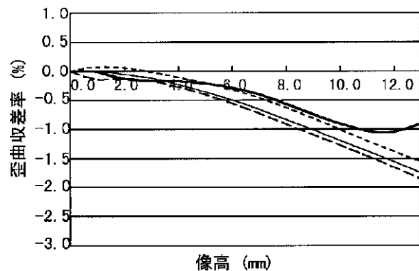
各撮影距離ごとの歪曲収差率の分布 (%)
