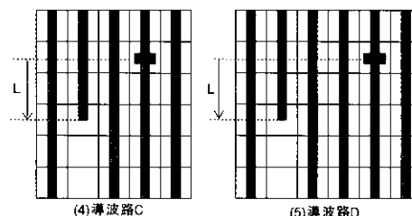
(4) 導波路C
