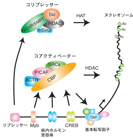
図 1. 転写制御における仲介因子の役割
