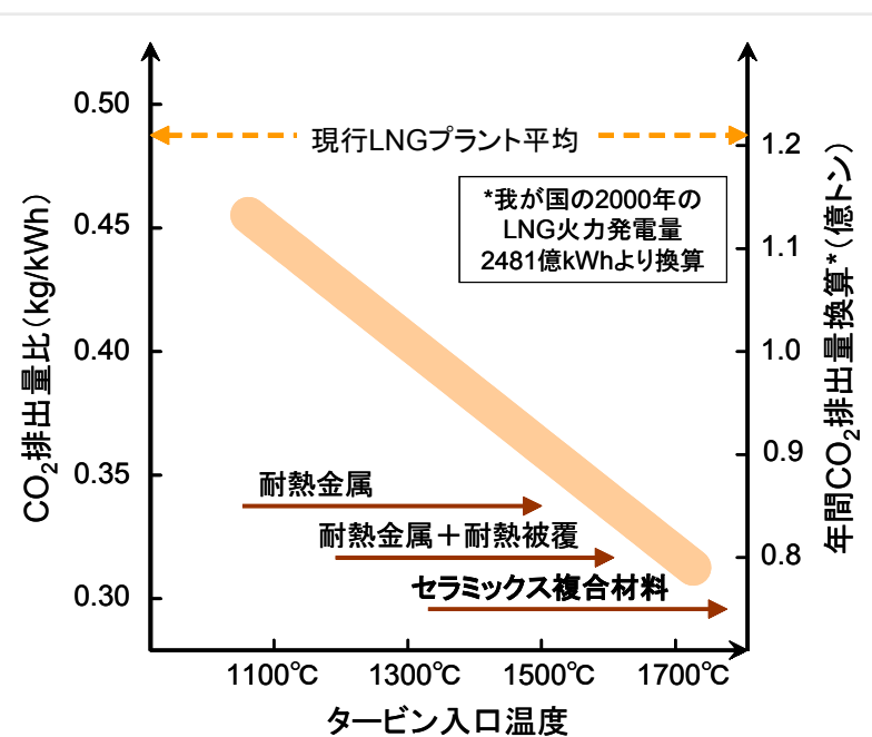
図1： 発電用ガスタービンへの超耐熱機能構造材料の適用による、LNG火力プラントからの二酸化炭素排出量削減への効果。超耐熱材料の開発は、その他のエネルギーシステム（ガス化石炭、ハイブリッド燃料電池、未利用化石燃料、第IV世代原子力、等）への適用を通じて、環境負荷低減に大きく寄与する。
