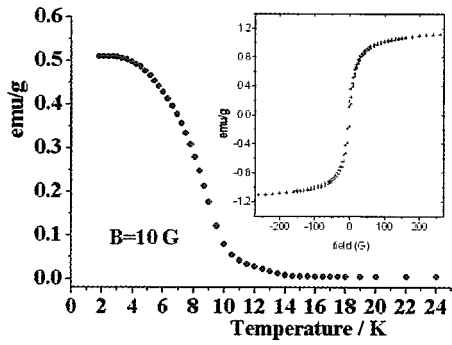
図3. BaMn 2 Ge 4 固体の磁気物性
