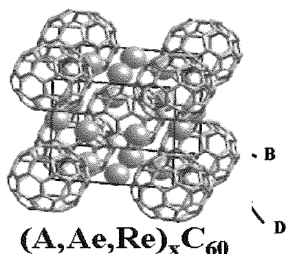
図1. C 60 多面体クラスタ結晶
