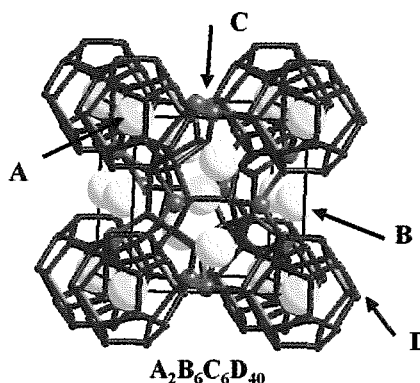
図2. Si/Ge多面体クラスタ結晶
